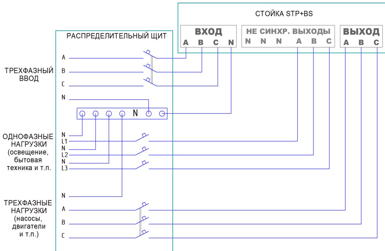
Рисунок 1. Рекомендуемая схема подключения Стойки STP+BS к сети.
